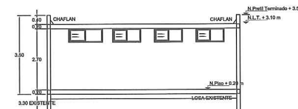
CORTE B - B' TALLER O SALON BODEGA
