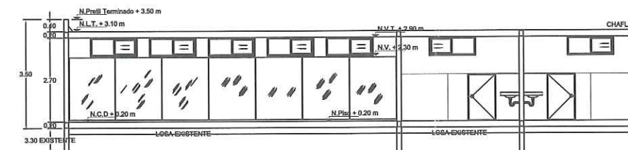
CORTE A - A' SALON CON PISO DE DUELA Y BAÑOS
