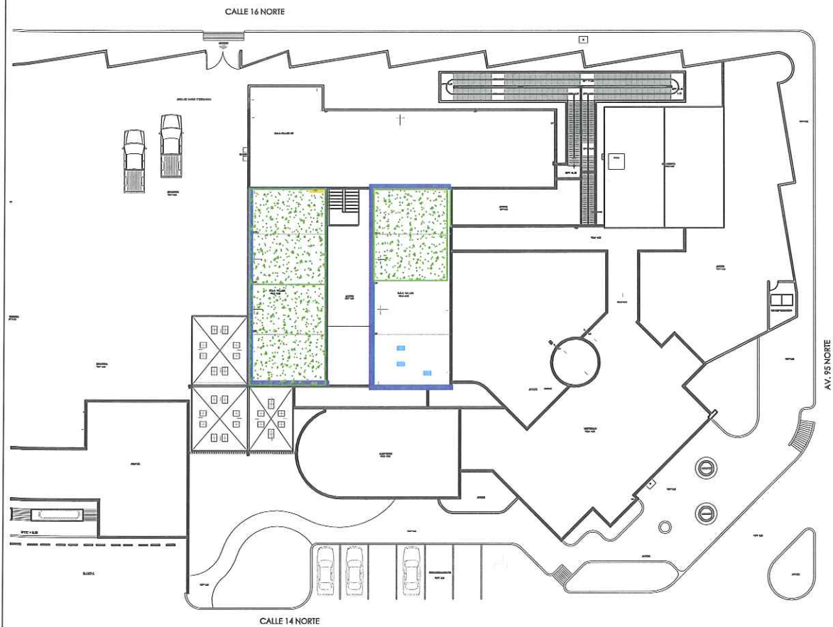
PLANO DE DEMOLICION Y RETIROS
