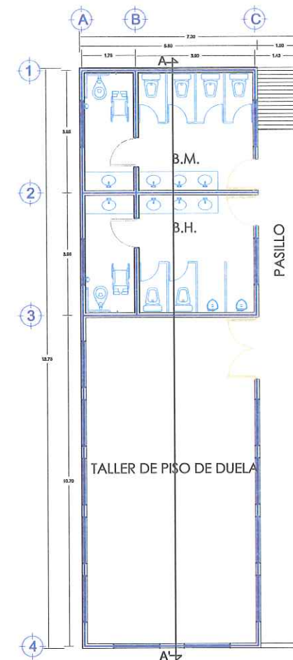
PLANTA ARQUITECTONICA TALLER CON PISO DE DUELA Y BAÑOS
